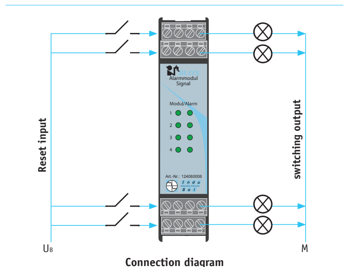
INBLOX® Alarm module
