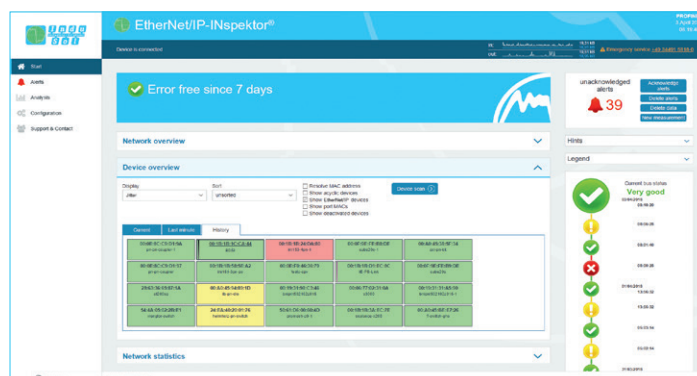
Web interface
